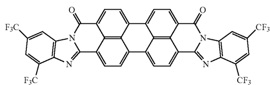
(P-1b)
