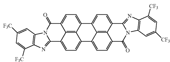
(P-1a)
