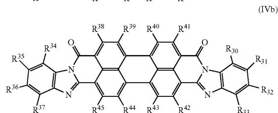
(IVb)
