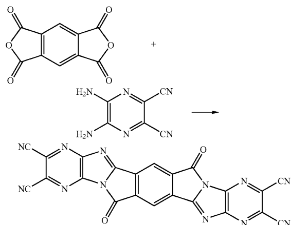
(A-3a)
