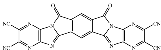
(A-3b)
